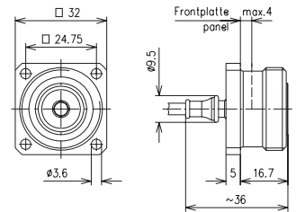
7-16 Gehäusekuppel mit Viereckflansch 7-16 fixed socket with four hole mounting flange
